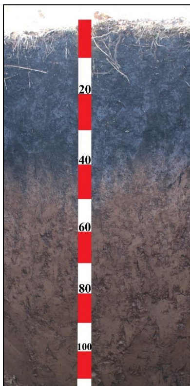
Рисунок 10.8 – Чернозём оподзоленный
