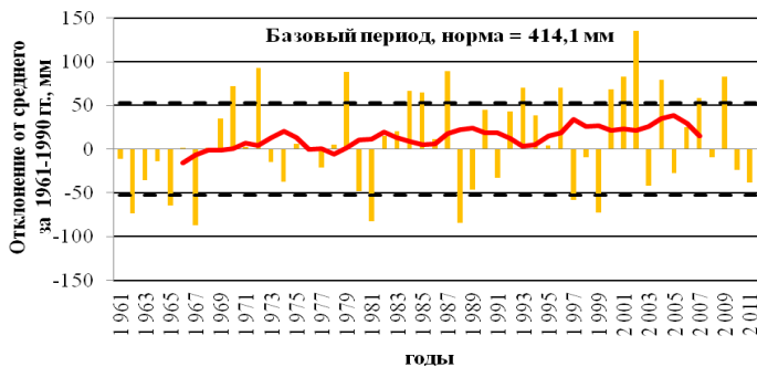
Рис. 6. Временной ход аномалий сумм атмосферных осадков на территории юго-востока Западной Сибири за период 1961–2012 гг.
