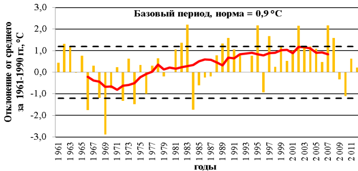
Рис. 1. Временной ход аномалий средней годовой температуры воздуха на территории юго-востока Западной Сибири за период 1961–2012 гг.
