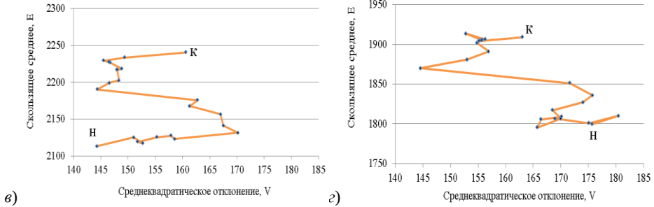
Рис. 4 – EV-диаграммы изменений центров распределения и разброса P_{5,10} (а, б) и \Sigma T_{5,10} (в, з) для скользящих 30-летних периодов с 1990 по 2012 гг. на территории юго-востока Западной Сибири (точка H – соответствует состоянию климата за 1961–1990 гг., а точка K – состояние климата за 1983–2012 гг.)
