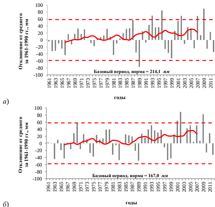
Рис. 7. Временной ход аномалий R_{5,10} (а, б) на территории юго-востока Западной Сибири
