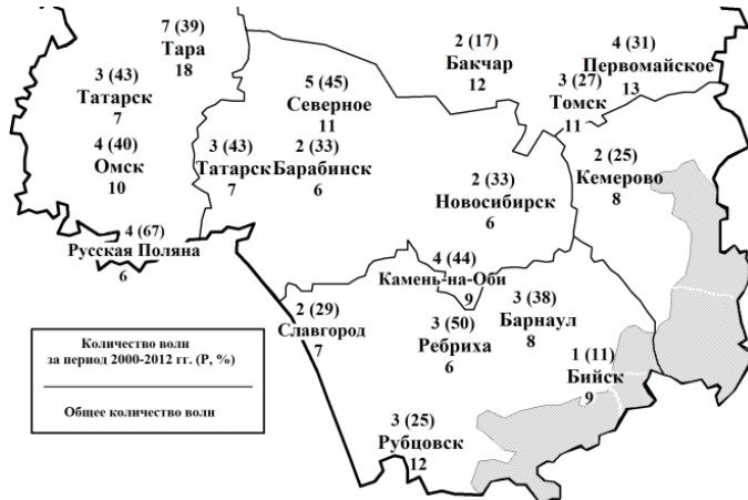
Рис. 12 – Карта-схема распределения повторяемости волн тепла на территории юго-востока Западной Сибири в критический период жизни ранних яровых зерновых культур (Р – повторяемость волн за период 2000–2012 гг., %)
