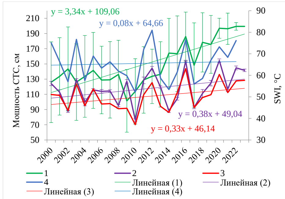
Рисунок 17 – Динамика значений 1) мощности СТС, 2) SWI LST , 3) SWI M , 4) SWI LSTM на участке №2 за период с 2000 по 2023 гг. (в виде пределов погрешностей указаны значения стандартного отклонения)
