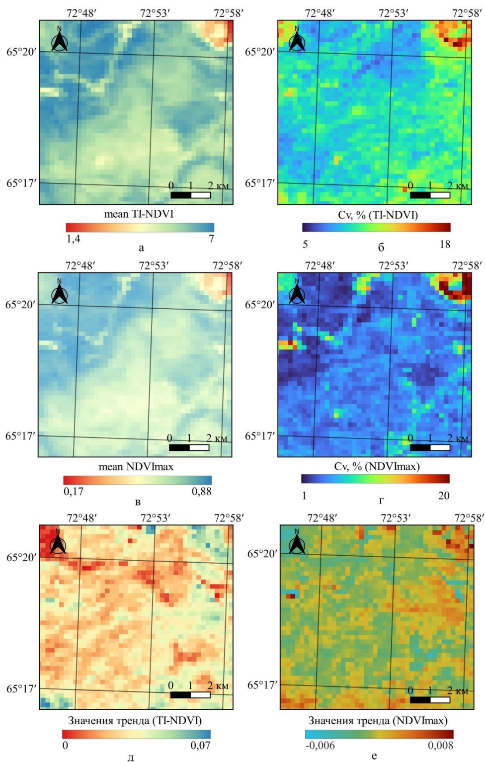
Рисунок 32 – Карты показателей вегетационного индекса на участке №2 за период с 2000 по 2023 гг.: а) осредненное значение TI-NDVI, б) коэффициент вариации (Cv) TI-NDVI, в) осредненное значение NDVI max , г) коэффициент вариации (Cv) NDVI max , д) значения линейного тренда TI-NDVI, е) значения линейного тренда NDVI max
