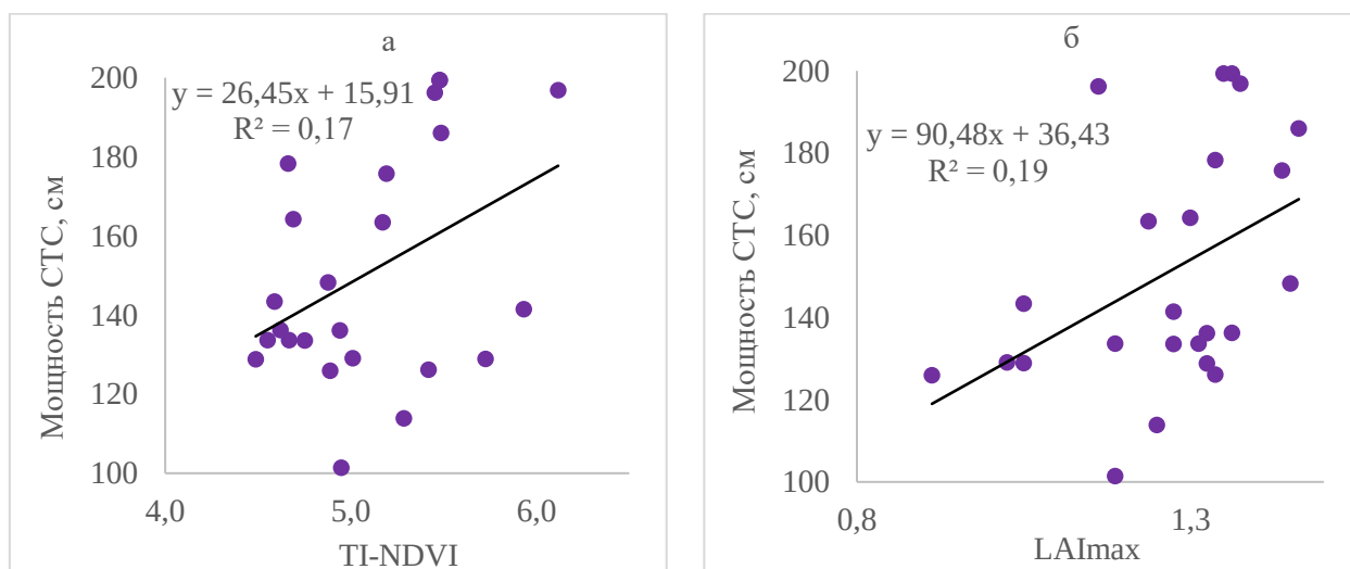
Рисунок 46 – Взаимосвязь мощности СТС мёрзлых торфяников с а) TI-NDVI б) LAI_{max} на участке №2 за период с 2000 по 2023 гг.
