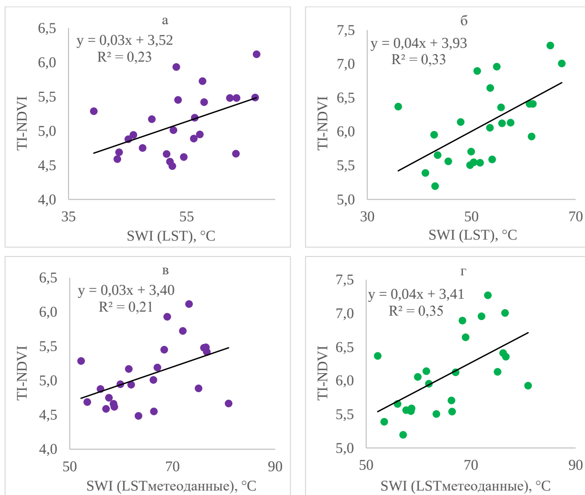
Рисунок 45 – Взаимосвязь SWI_{LST} и SWI_{LSTM} с TI-NDVI а), в) торфяников и б), г) лесов и редколесий на участке №2 за период с 2000 по 2023 гг.
