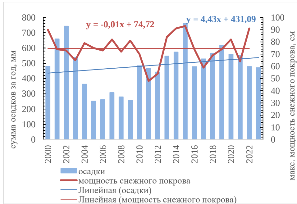
Рисунок 4 – Межгодовые изменения суммы осадков за год и максимальной мощности снежного покрова по данным метеостанции Юильск
