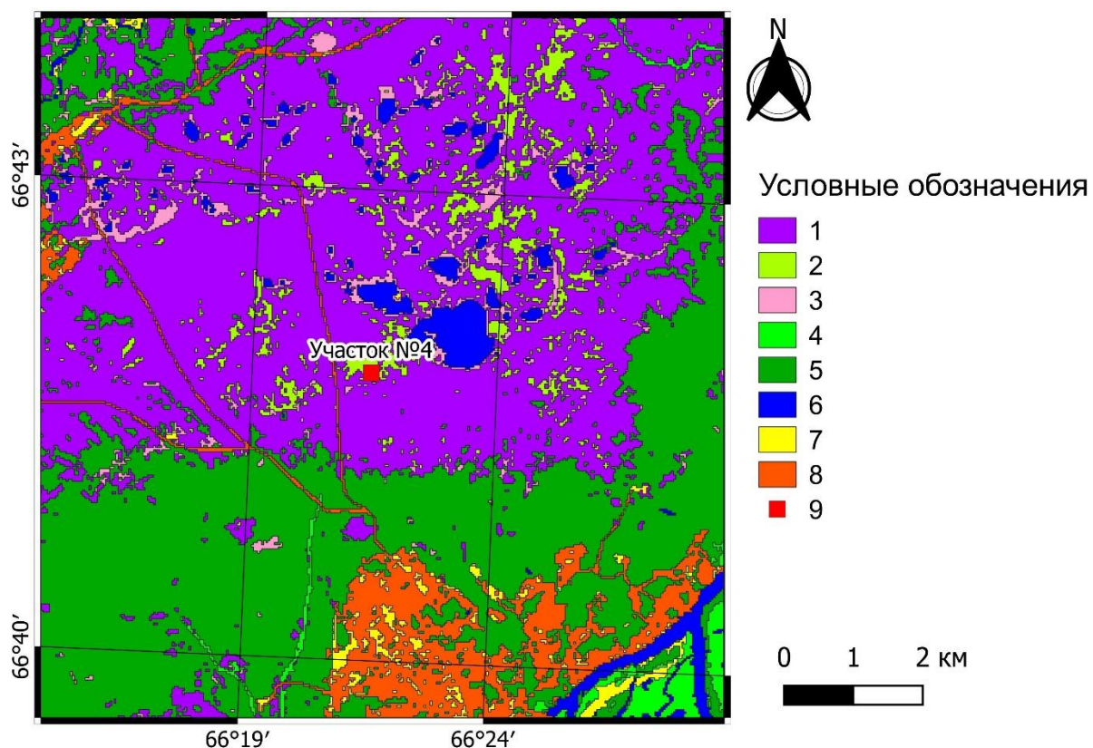
Рисунок 2.4 – Участок №4 (стационар Лабытнанги). Алгоритм “Minimum Distance”.
