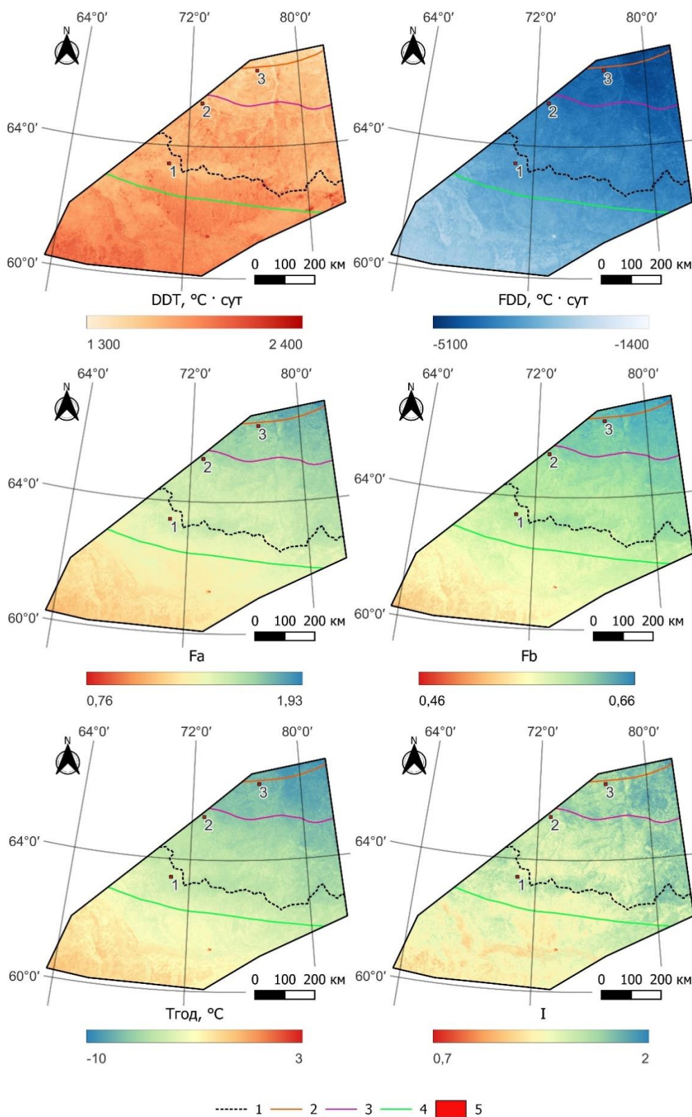
Рисунок 27 – Карты средних значений климатических параметров и индексов центральной части севера Западной Сибири за период 2014–2023 гг. 1 – граница субъектов Российской Федерации (ХМАО и ЯНАО); южные границы зон распространения ММП: 2 – сплошной, 3 – прерывистой, 4 – островной; 5 – участки исследования
