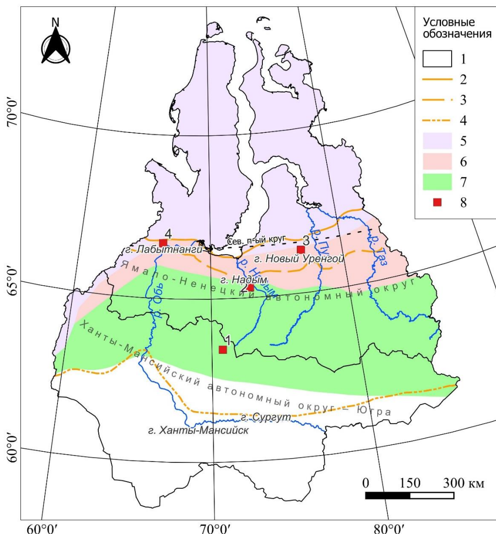
Рисунок 1 – Район исследований. 1 – административно-территориальные границы ЯНАО и ХМАО – Югры; 2–4 – границы геоботанических зон и подзон по (Ильина и др., 1985): 2 – лесотундры, 3 – северной тайги, 4 – средней тайги; 5–7 – зоны распространения ММП по (Геокриологическая карта СССР..., 1991): 5 – сплошная, 6 – прерывистая, 7 – островная и редкоостровная; 8 – участки исследования: 1 – участок №1 (природный парк «Нумто»), 2 – участок №2 (Надымский стационар), 3 – участок №3 (Южный Уренгой), 4 – участок №4 (Лабытнанги)
