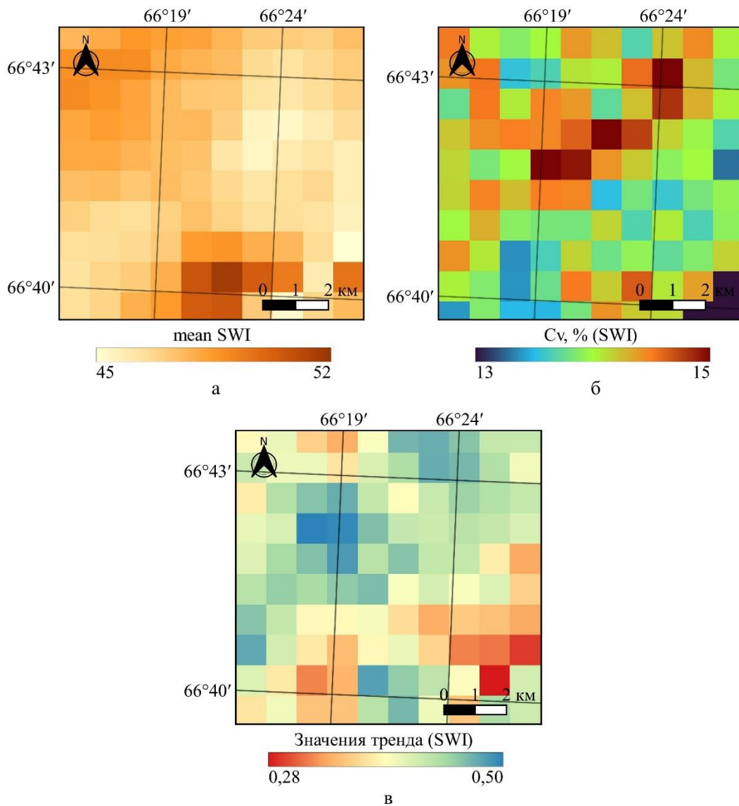
Рисунок 23 – Карты-схемы показателя SWI LST на участке №4 за период с 2000 по 2023 гг.: а) осредненное значение SWI LST , б) коэффициент вариации (Cv) SWI LST , в) значения линейного тренда SWI LST
