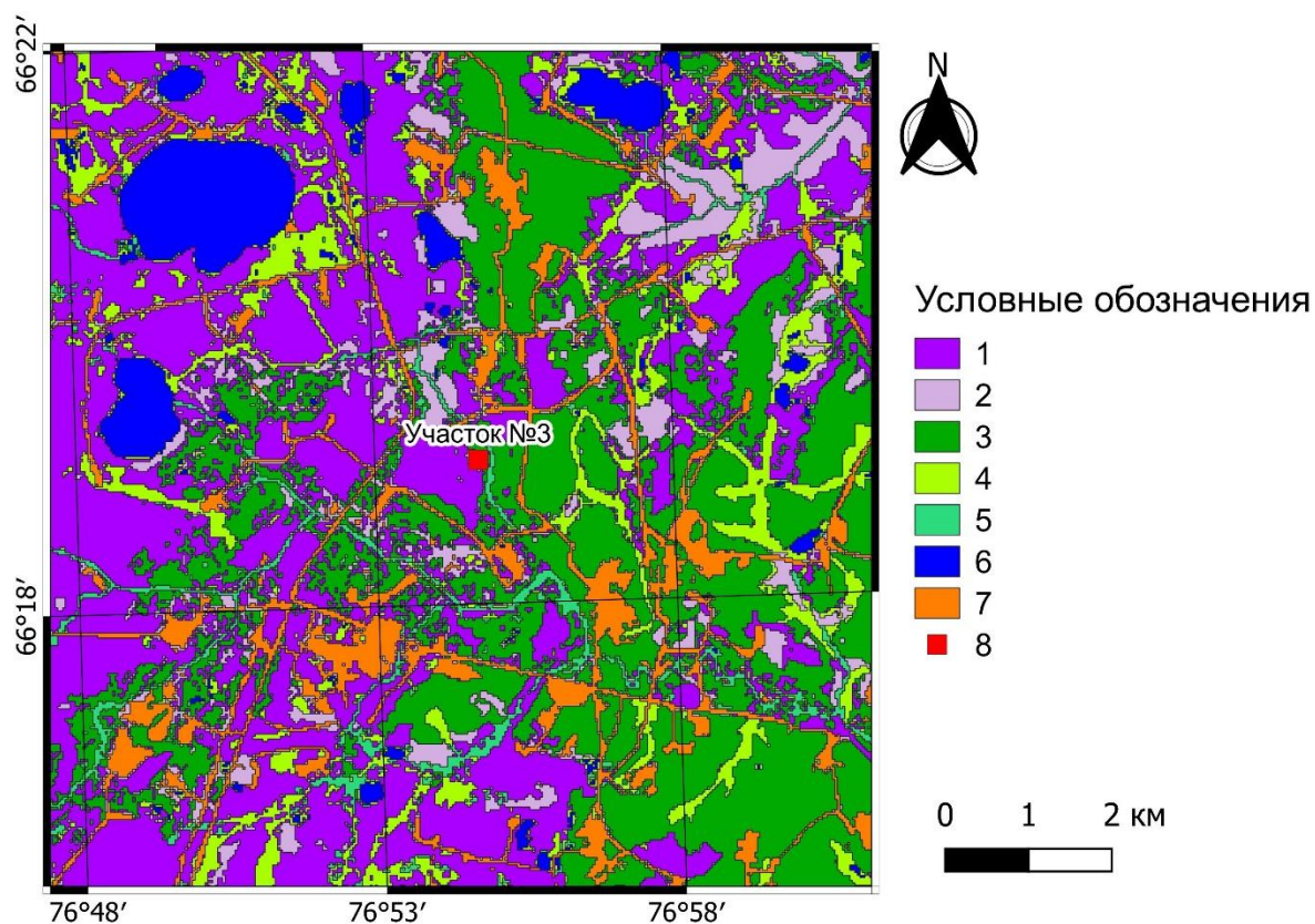
Рисунок 2.3 – Участок №3 (Южный Уренгой). Алгоритм “Minimum Distance”.
