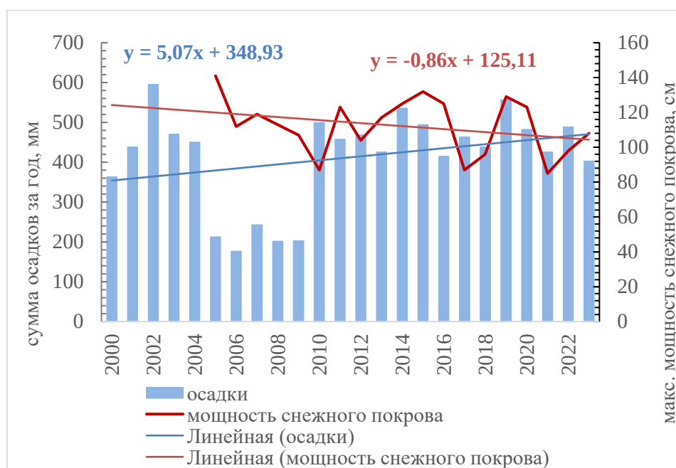
Рисунок 8 – Межгодовые изменения суммы осадков за год и максимальной мощности снежного покрова по данным метеостанции Новый Уренгой
