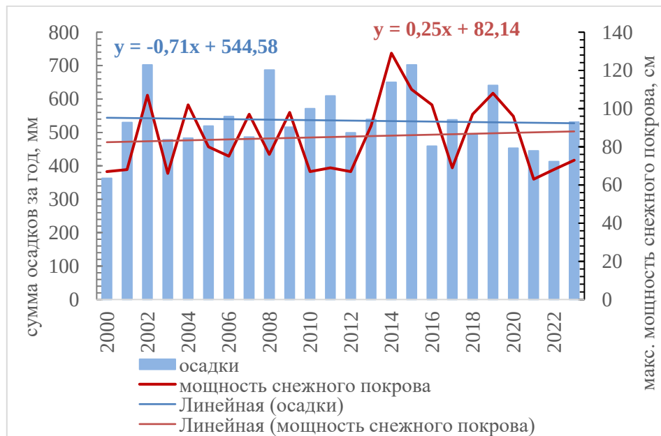
Рисунок 6 – Межгодовые изменения суммы осадков за год и максимальной мощности снежного покрова по данным метеостанции Надым
