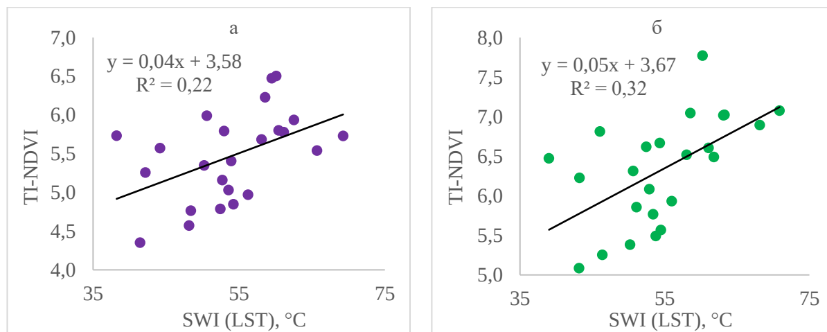
Рисунок 44 – Взаимосвязь TI-NDVI с SWI_{LST} а) торфяников и б) лесов и редколесий на участке №1 за период с 2000 по 2023 гг.
