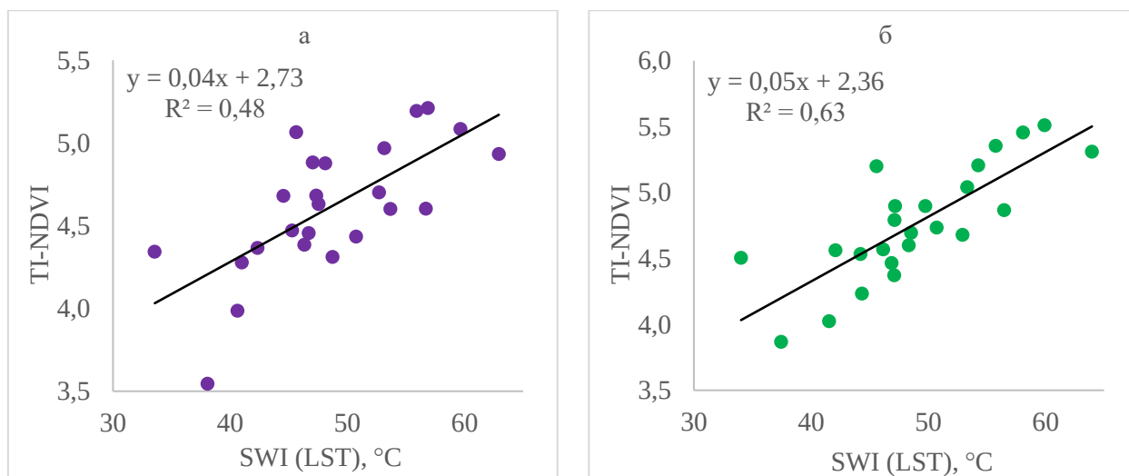
Рисунок 47 – Взаимосвязь TI-NDVI с SWI_{LST} а) торфяников и б) лесов и редколесий на участке №3 за период с 2000 по 2023 гг.
