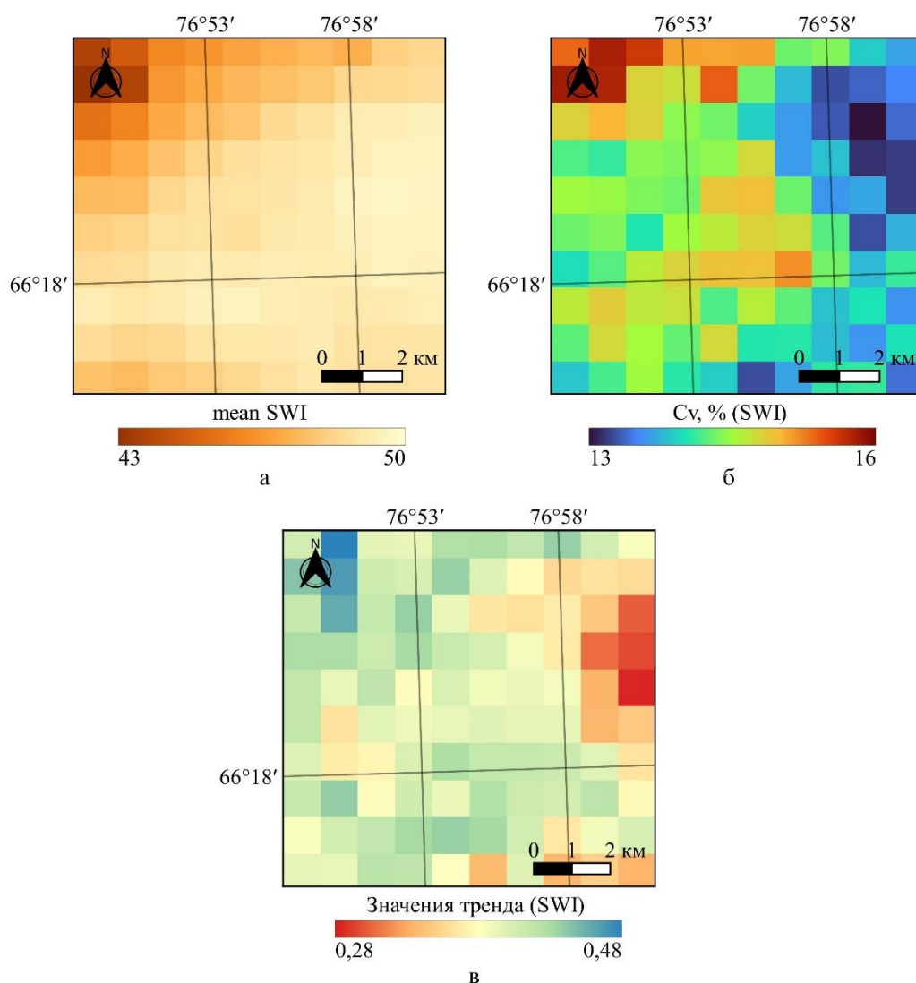
Рисунок 19 – Карты-схемы показателя SWI LST на участке №3 за период с 2000 по 2023 гг.: а) осредненное значение SWI LST , б) коэффициент вариации (Cv) SWI LST , в) значения линейного тренда SWI LST
