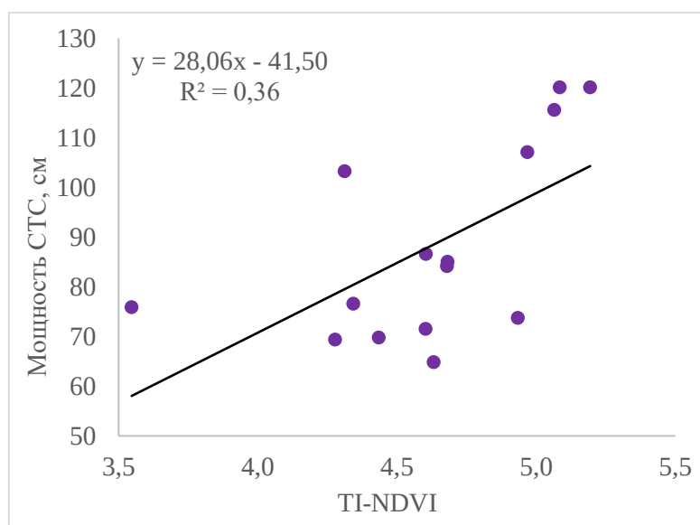
Рисунок 48 – Взаимосвязь мощности СТС мёрзлых торфяников с TI-NDVI на участке №3 за период с 2008 по 2022 гг.
