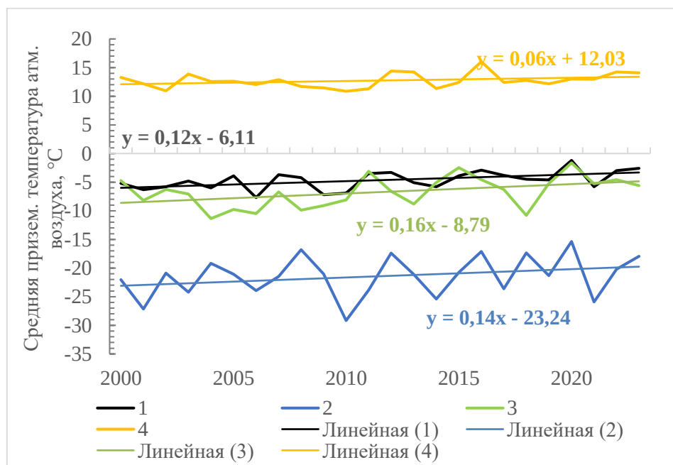
Рисунок 9 – Межгодовые изменения средних значений приземной температуры атмосферного воздуха по данным метеостанции Салехард за: 1) год; 2) зимний период, 3) весенний период, 4) летний период
