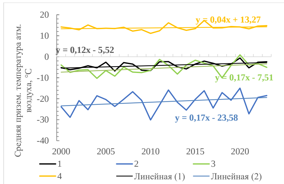
Рисунок 5 – Межгодовые изменения средних значений приземной температуры атмосферного воздуха по данным метеостанции Надым за: 1) год; 2) зимний период, 3) весенний период, 4) летний период
