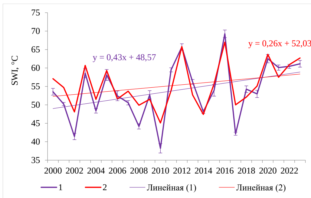
Рисунок 13 – Динамика значений 1) SWI_{LST} , 2) SWI_M мёрзлых торфяников на участке №1 за период с 2000 по 2023 гг. (в виде пределов погрешностей указаны значения стандартного отклонения)
