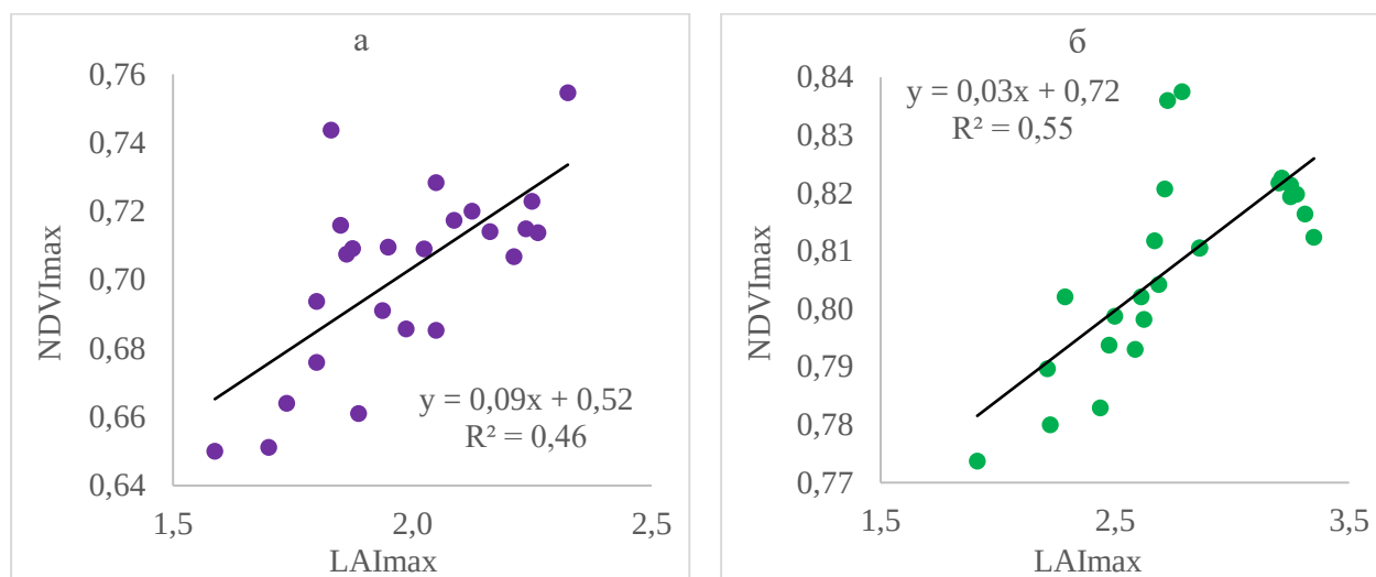
Рисунок 42 – Взаимосвязь между LAI_{max} и NDVI_{max} на участке №4 за период с 2000 по 2023 гг.: а) торфяники, б) лес
