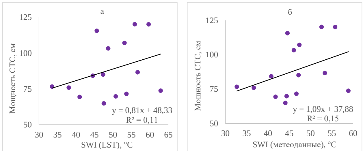
Рисунок 22 – Взаимосвязь мощности CTC мёрзлых торфяников с а) SWI_{LST} и б) SWI_M на участке №3 за период с 2008 по 2022 гг.
